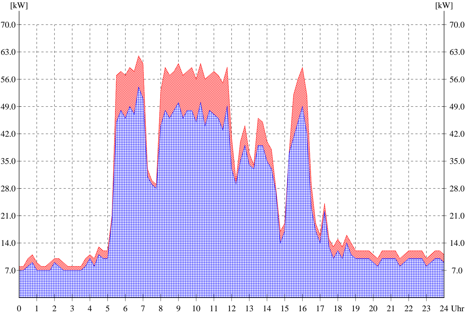
Diagramm Last-Leerlauf für den 02.12.2002
